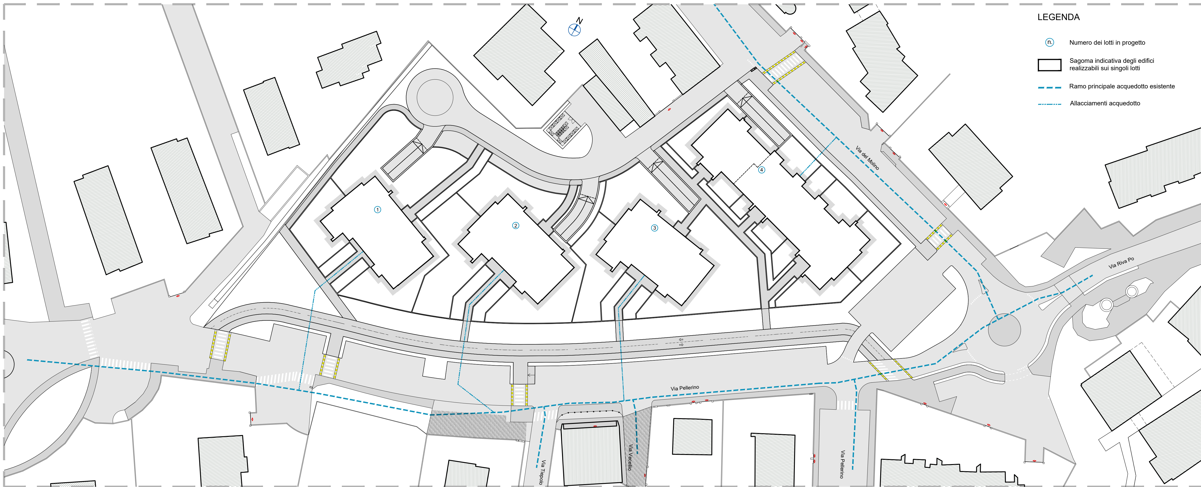
PLANIMETRIA GENERALE RETE ACQUEDOTTO ESISTENTE E ALLACCIAMENTI - SCALA 1:500
