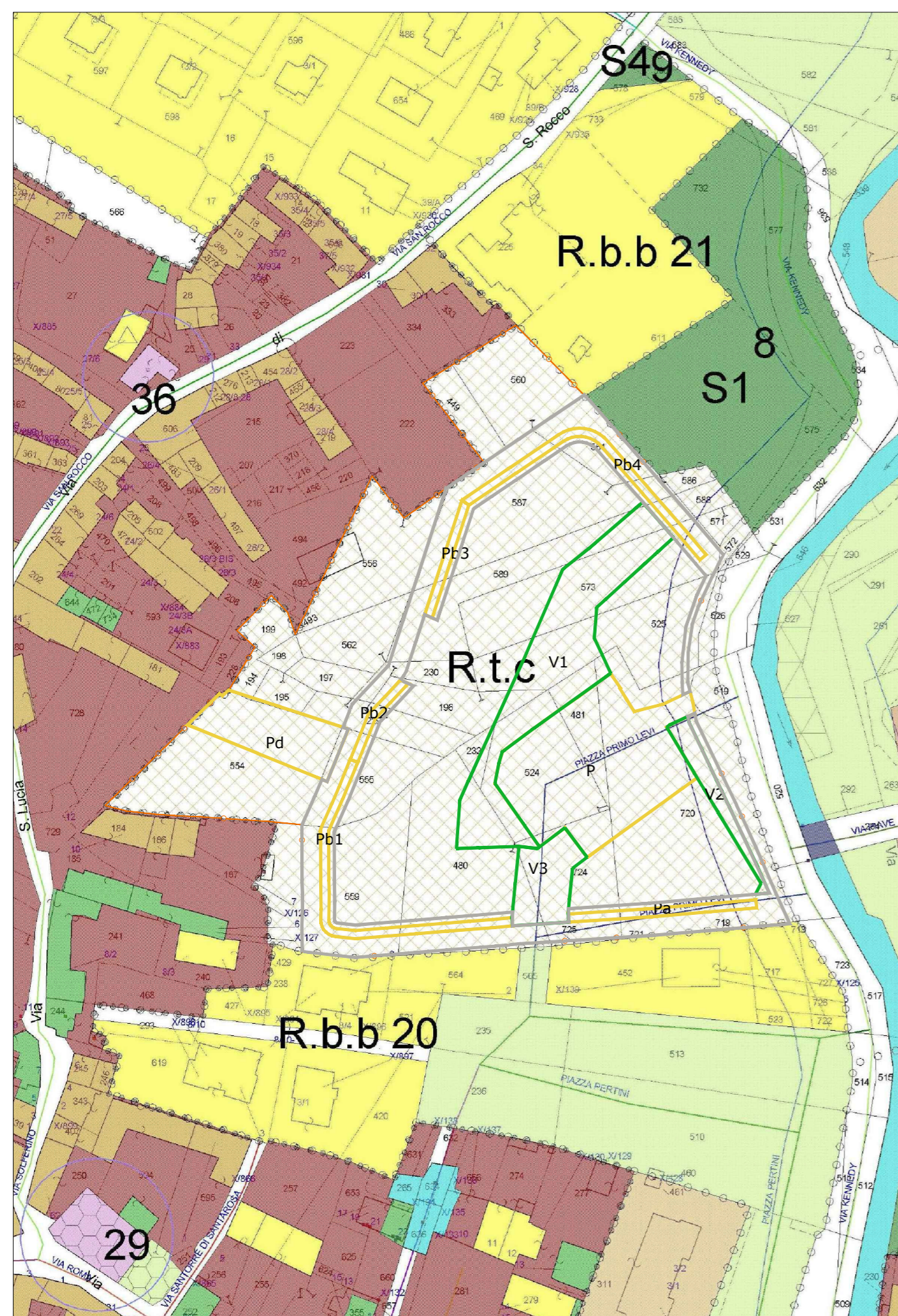
PLANIMETRIA SCALA 1:1500
