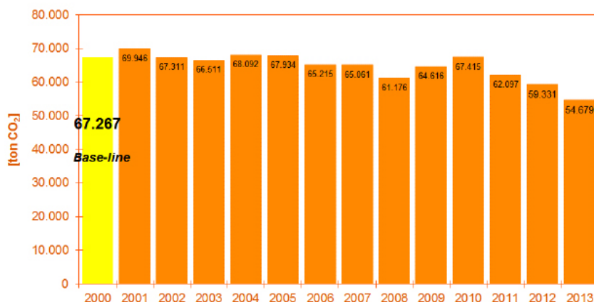
La definizione della BEI - evoluzione delle emissioni assolute di CO 2 (industria e agricoltura esclusi)
