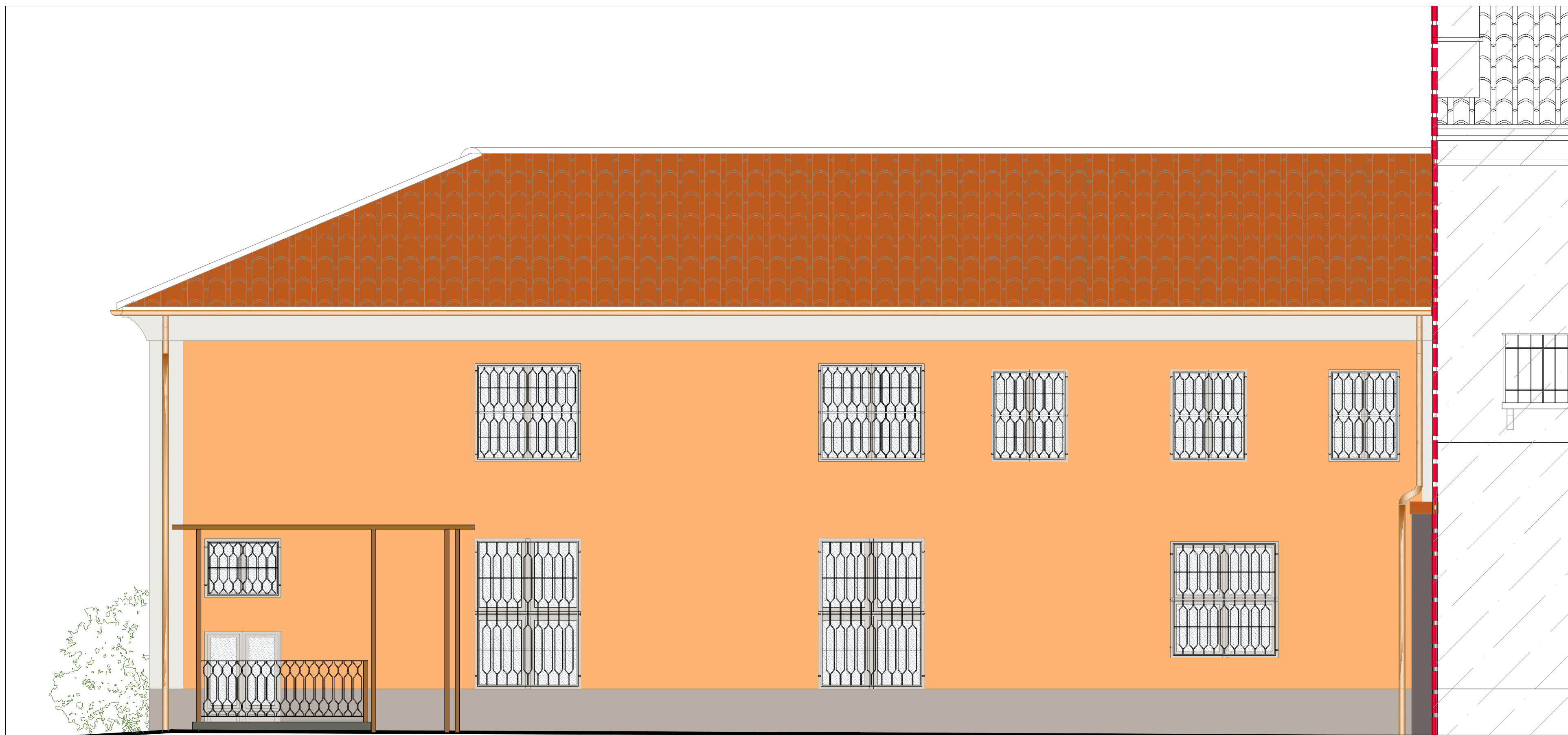
PROSPETTO POSTERIORE C (scala 1:50)
