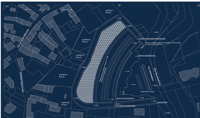
- PLANIMETRIA GENERALE DEL PROGETTO DEL COMUNE DI PIOSSASCO, PIANA A QUOTA +1.00, SCALA 1:1000
