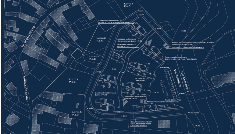
- PLANIMETRIA GENERALE DEL PROGETTO DEL COMUNE DI PIOSSASCO, PIANA A QUOTA +10.00, SCALA 1:1000
