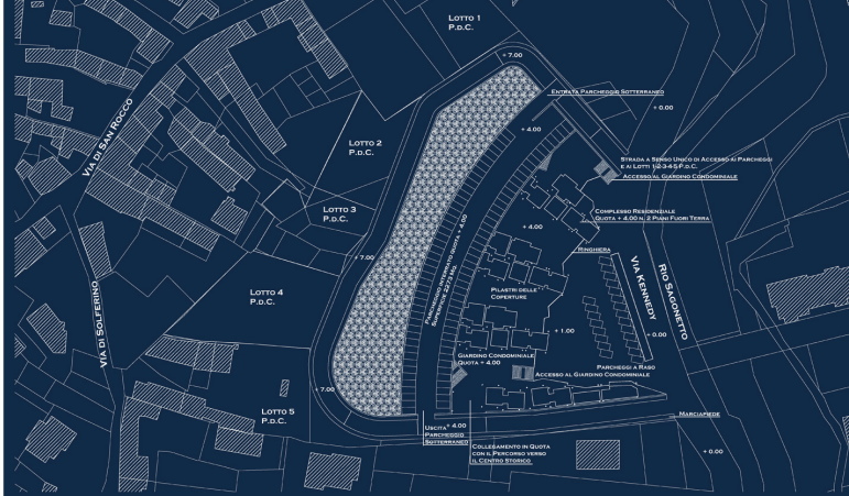
- PLANIMETRIA GENERALE DEL PROGETTO DEL COMUNE DI PIOSSASCO, PIANA A QUOTA +4.00, SCALA 1:1000
